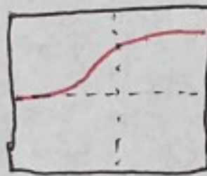
Sigmoide
