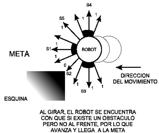
Figura 10: Utilización de más sonares.
