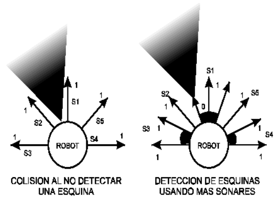
Figura 9: Detección de esquinas.
