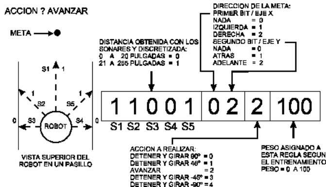
Figura 4: Creación de una regla.
