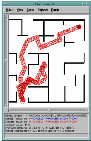
Figura 8: Ejemplo de navegación saliendo de trampas.
